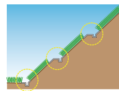
法面小段排水の施工例
